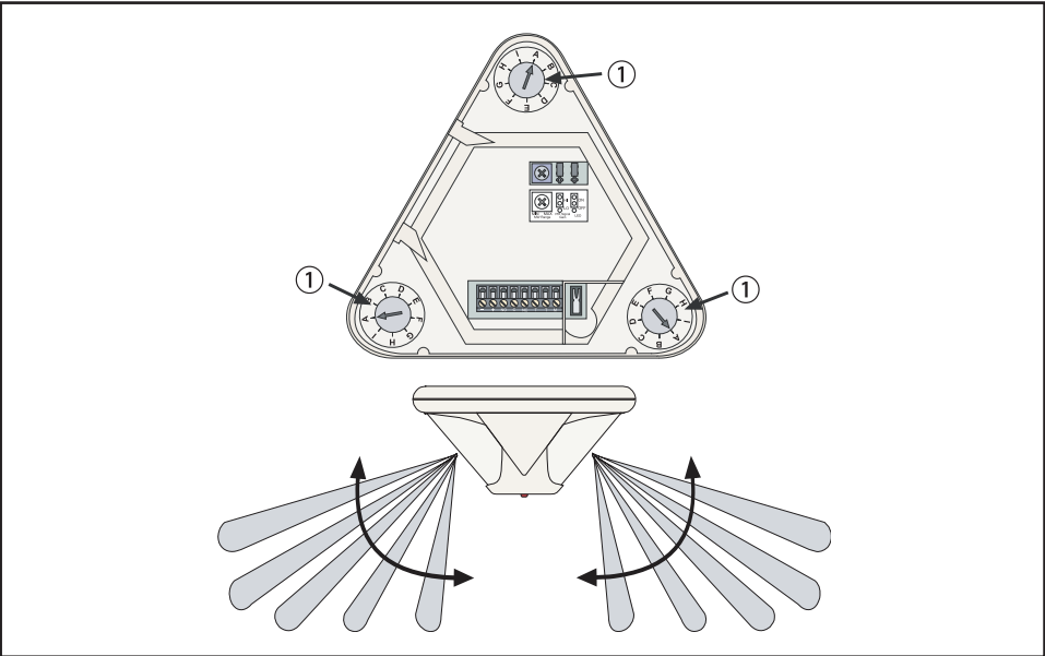
Figure 10.1 : diagrammes de couverture IRP et boutons de réglage vertical (1) Les zones IRP du DS939 sont divisées en trois groupes. Chacun de ces 3 groupes peut être réglé verticalement de façon indépendante afin de fournir la meilleure couverture dans une pièce. Pour des raisons de clarté, seulement deux diagrammes de couverture sont représentés. Voir Figure 10.1. Pour régler les modules optiques en fonction de la hauteur de montage du détecteur, reportez-vous au tableau 10.1. La portée affichée est la distance entre le détecteur et le bord extérieur du diagramme de couverture.
